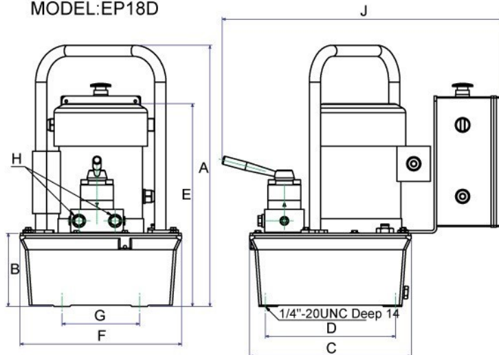
MODEL:EP18D
